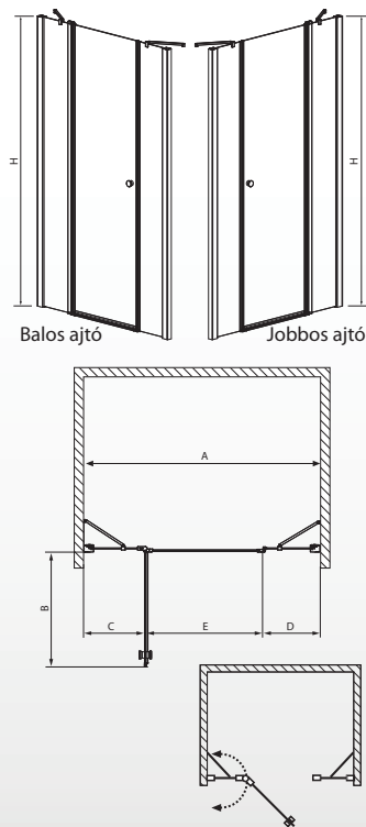
A képen balos zuhanyfal látható.
