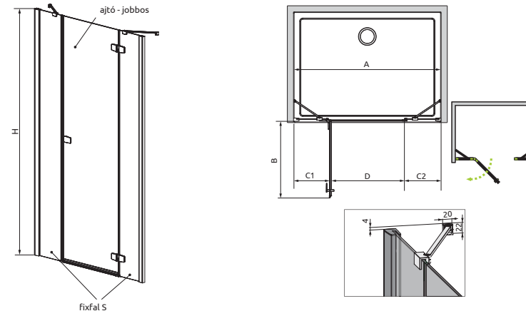
A rajzon jobb zuhanyajtó látható.
