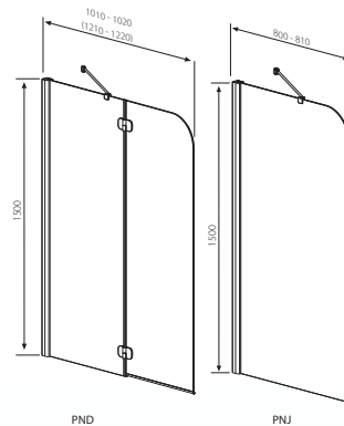
A rajzon balos kádparaván látható.
