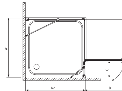
A rajzon balos zuhanykabin látható.
