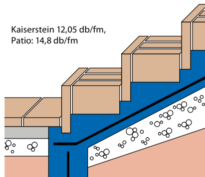
↑ lépcső kialakítás 4
